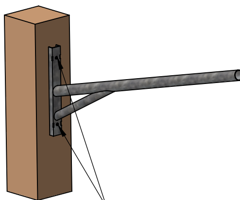
Fixation sur support par 2 boulons M14. - La distance entre 2 boulons sera réalisée selon la specification du client.
