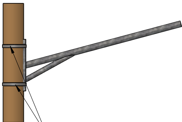
Fixation sur poteau par 2 feuillards
